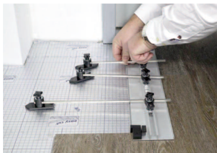
Abb 1. Grundplatte an der Belagskante anlegen
